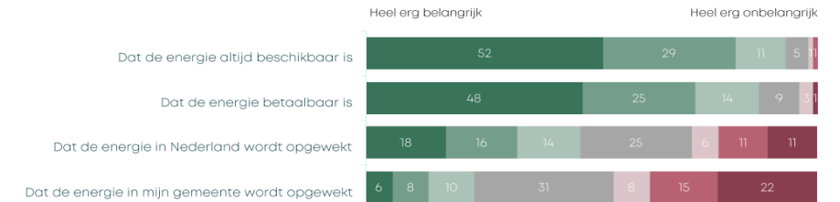
Stellingen opwekken en gebruik energie (%)
